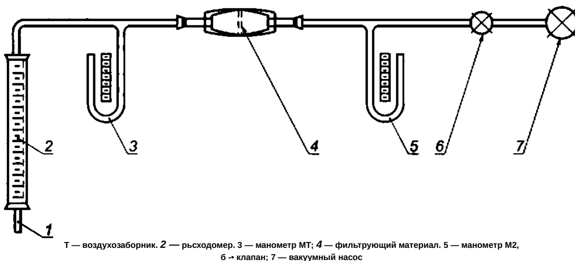
Рисунок С.1 — Прибор для измерения сопротивления воздуха
